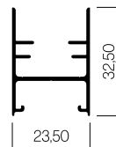
Perfil fijo 27 042098
