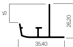
Guía Avant 031241
