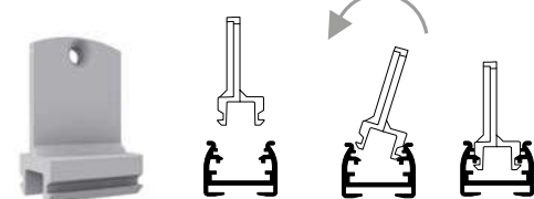
Soporte superior
