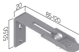
Jgo. soporte inferior
