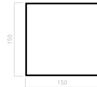
Pérgola sencilla y dúplex Columna P-150x150x2,5 mm ■ 023101
