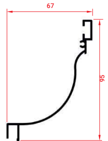
CANALÓN SUPERIOR | CHÉNEAU SUPÉRIEUR | UPPER GUTTER
