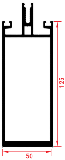
MONTANTE 125 | MONTANT 125 | UPRIGHT 125
