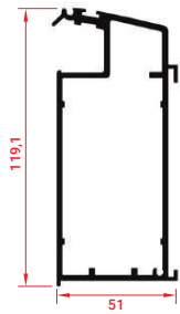
VIGA ESTRUCTURAL | LINTEAU AVANT RENFORCÉ | STRUCTURAL BEAM
