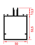
CANALÓN INFERIOR | CHÉNEAU INFÉRIEUR | BOTTOM GUTTER
