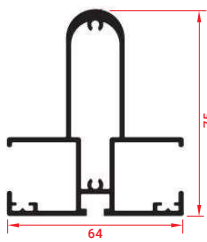
GUÍA 1 HOJAS | GUIDE 1 RAILS | GUIDE 1 SHEETS
