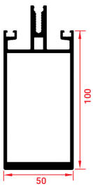
MONTANTE 100 | MONTANT 100 | UPRIGHT 100
