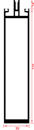
MONTANTE 225 | MONTANT 225 | UPRIGHT 225
