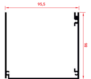
CANALÓN INFERIOR | CHÉNEAU INFÉRIEUR | BOTTOM GUTTER
