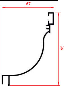
CANALÓN SUPERIOR | CHÉNEAU SUPÉRIEUR | UPPER GUTTER
