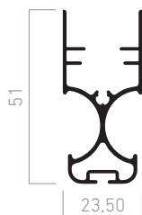
Perfil móvil 27 042096
